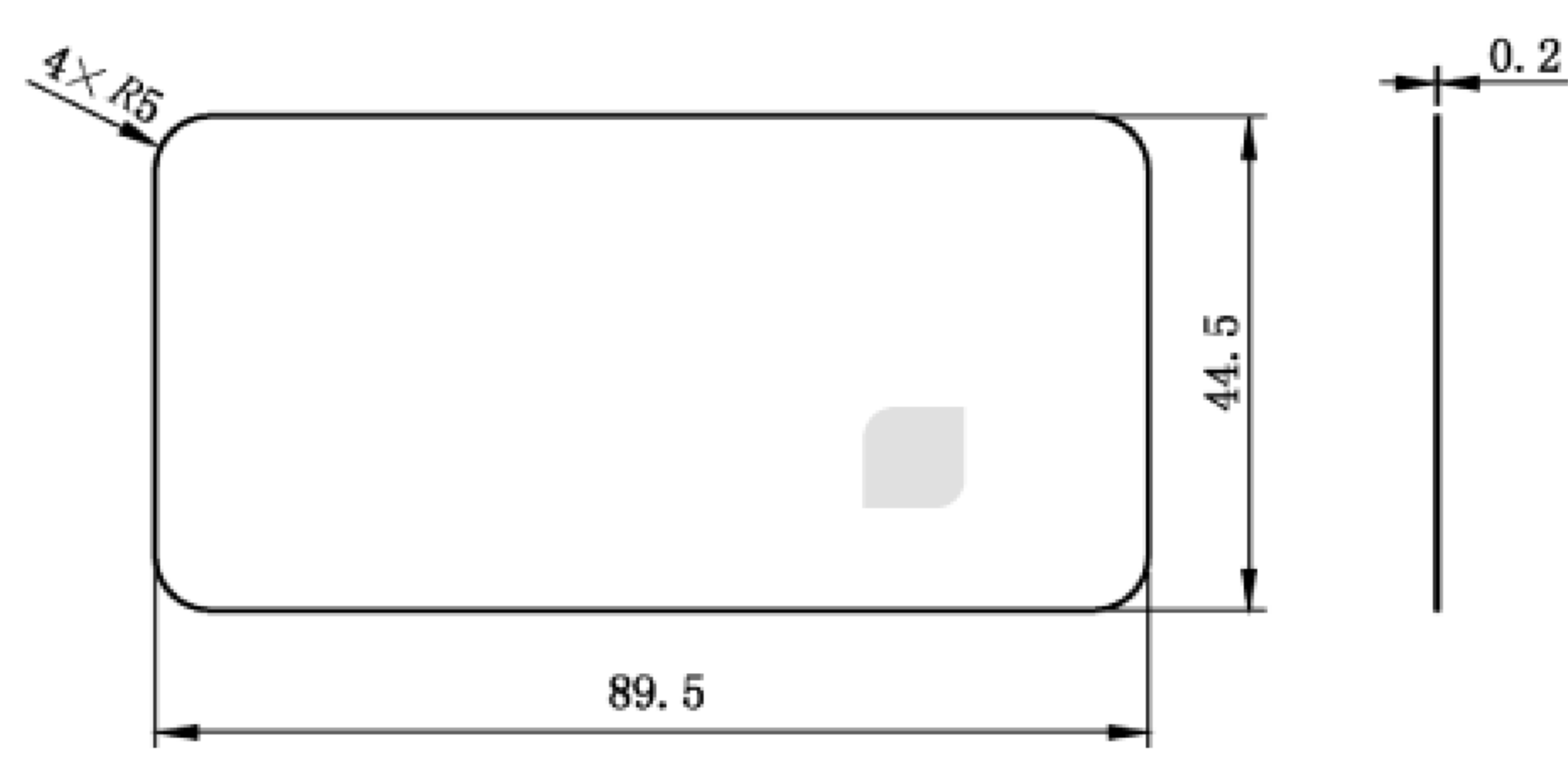
图 A.22 薄钢板
