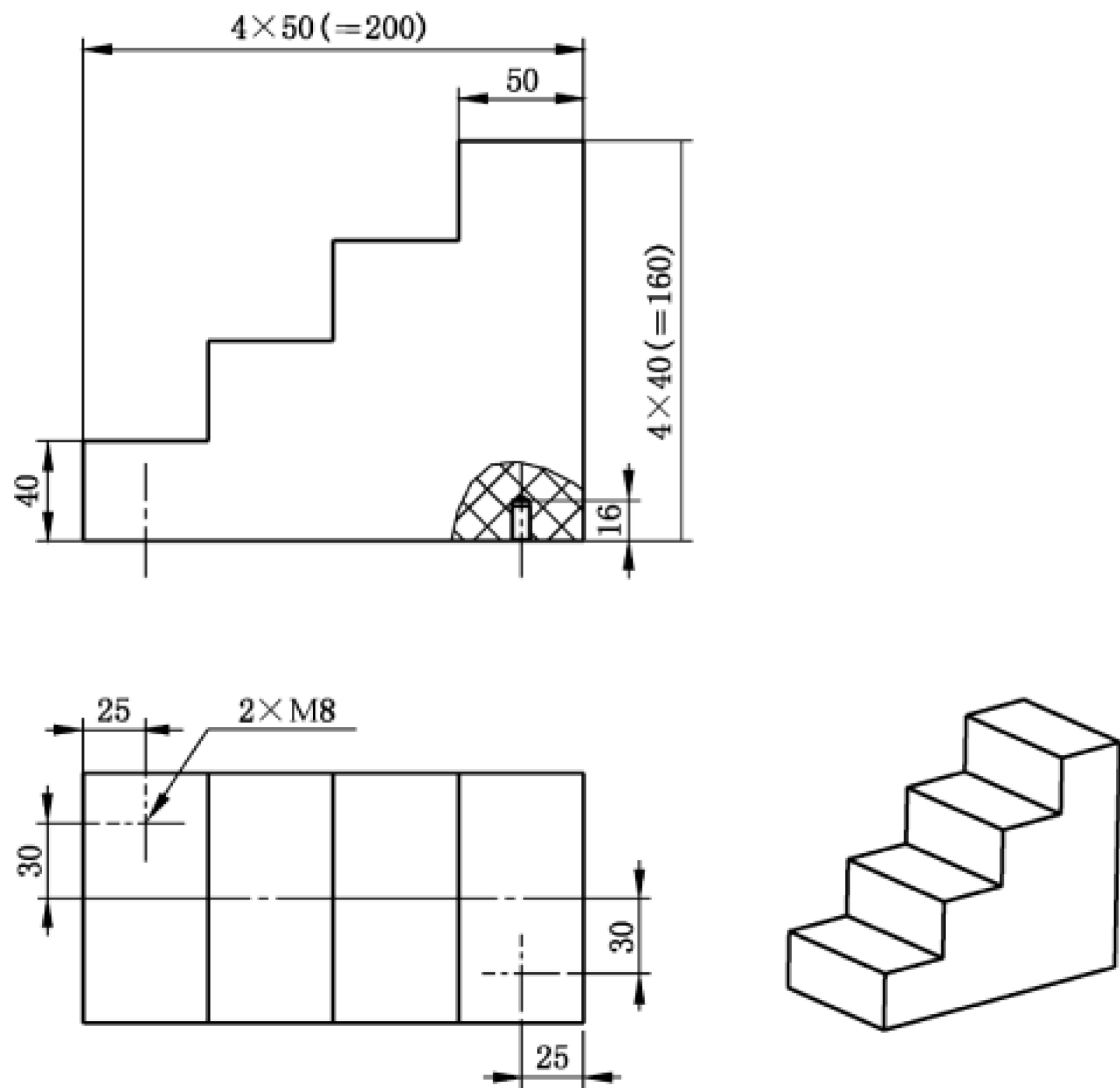
图 A.17 测试卡 4
