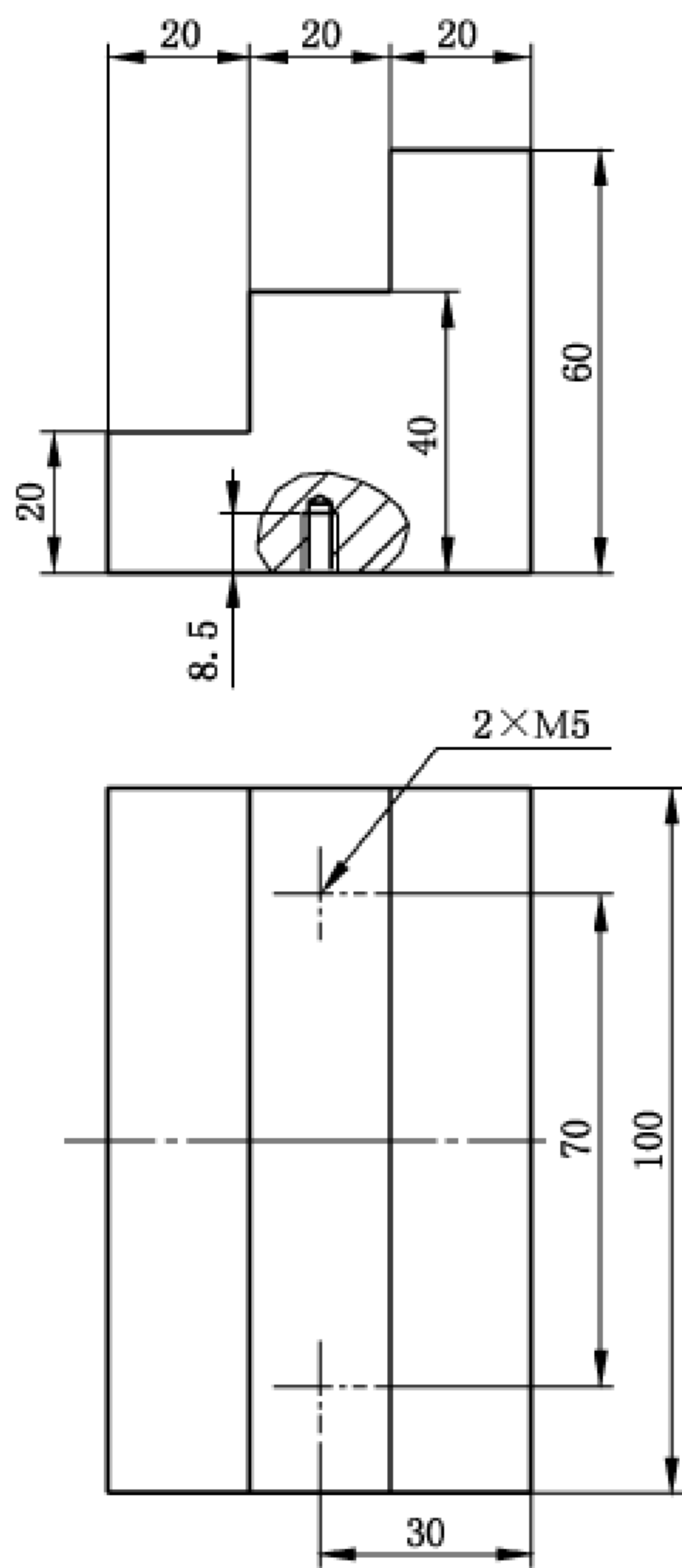
图 A.20 测试卡 5 厚合金铝阶梯
