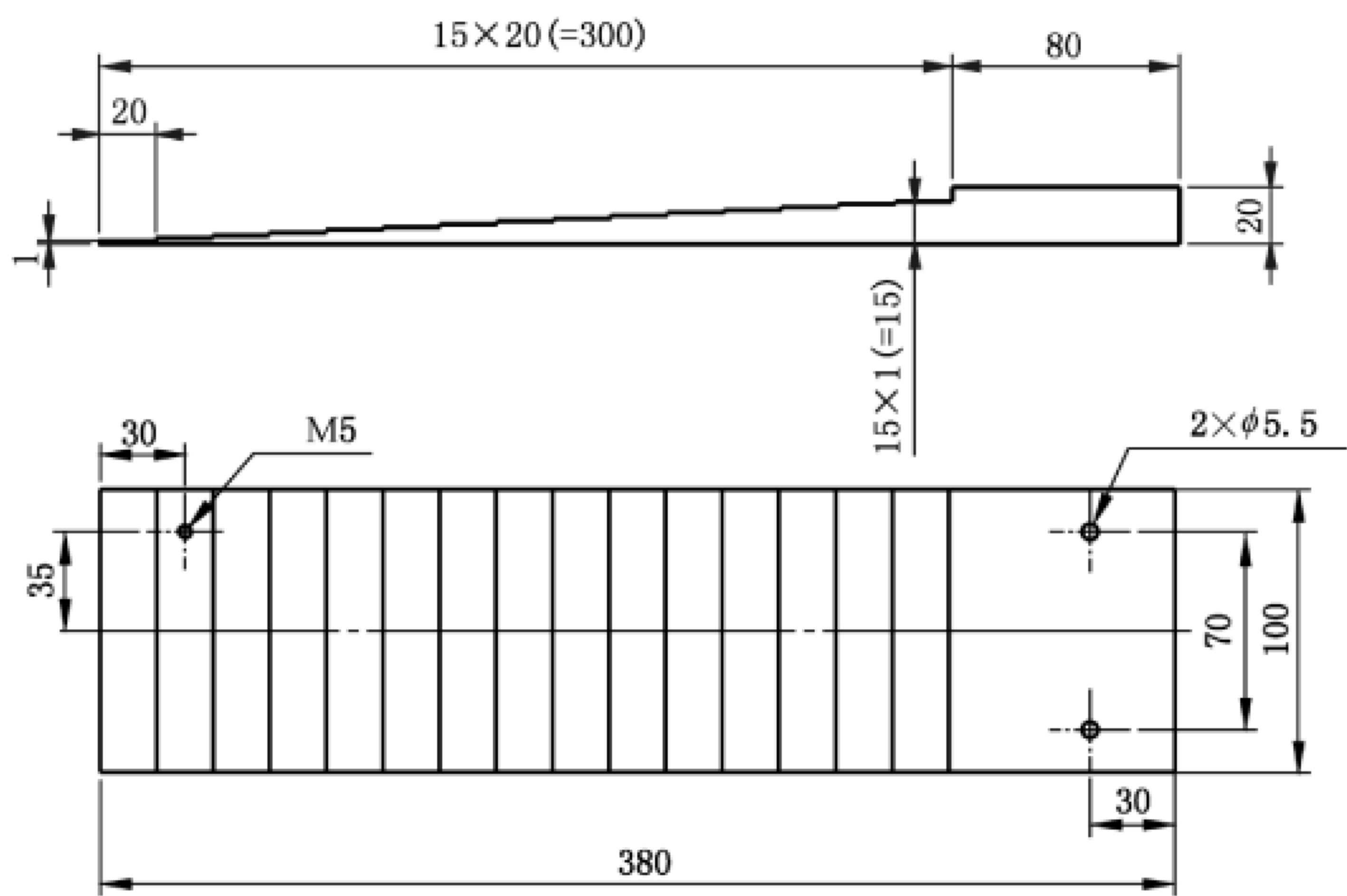
图 A.19 测试卡 5 薄合金铝阶梯
