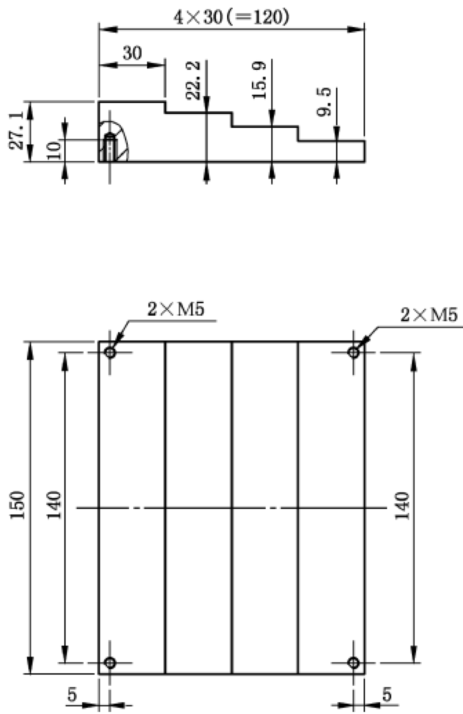
图 A.14 测试卡 2 合金铝阶梯
