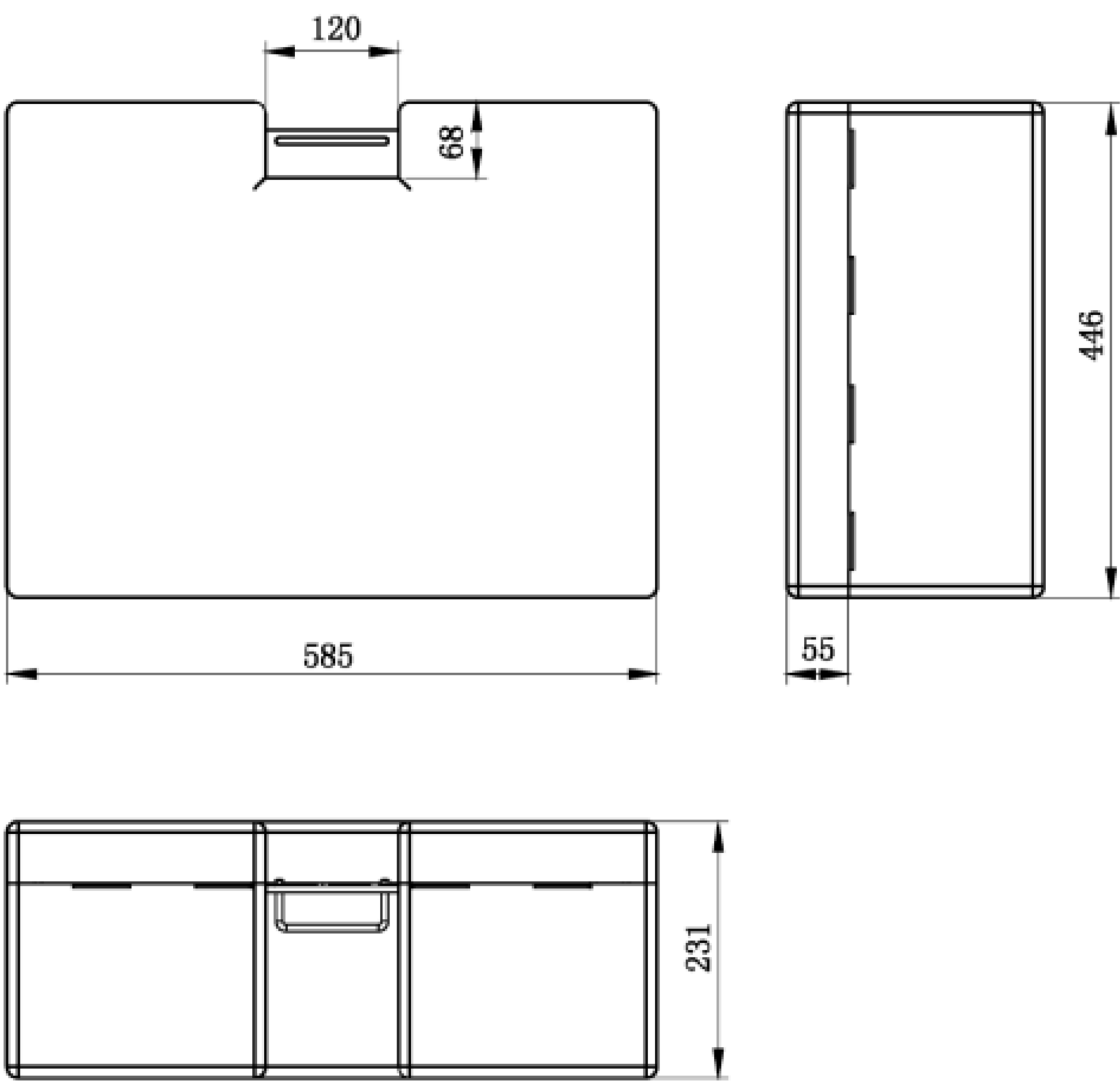
图 A.3 测试体 B 外形图
