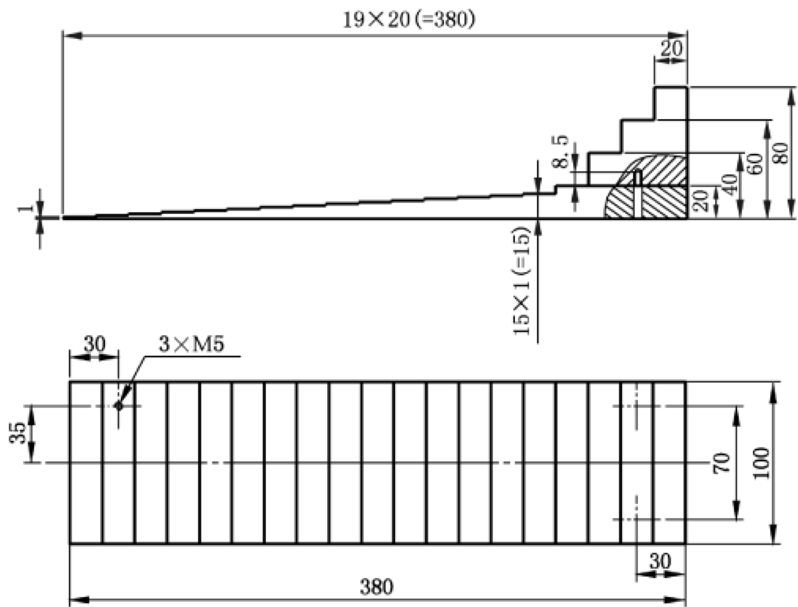
图 A.18 测试卡 5
