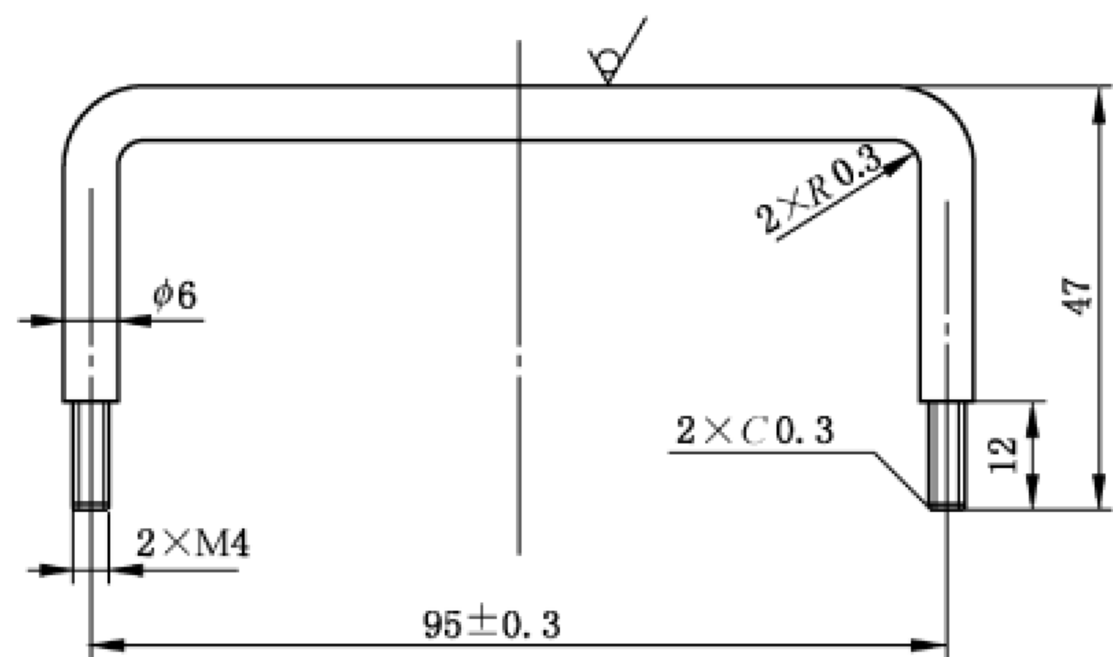
图 A.10 测试体 B 提手
