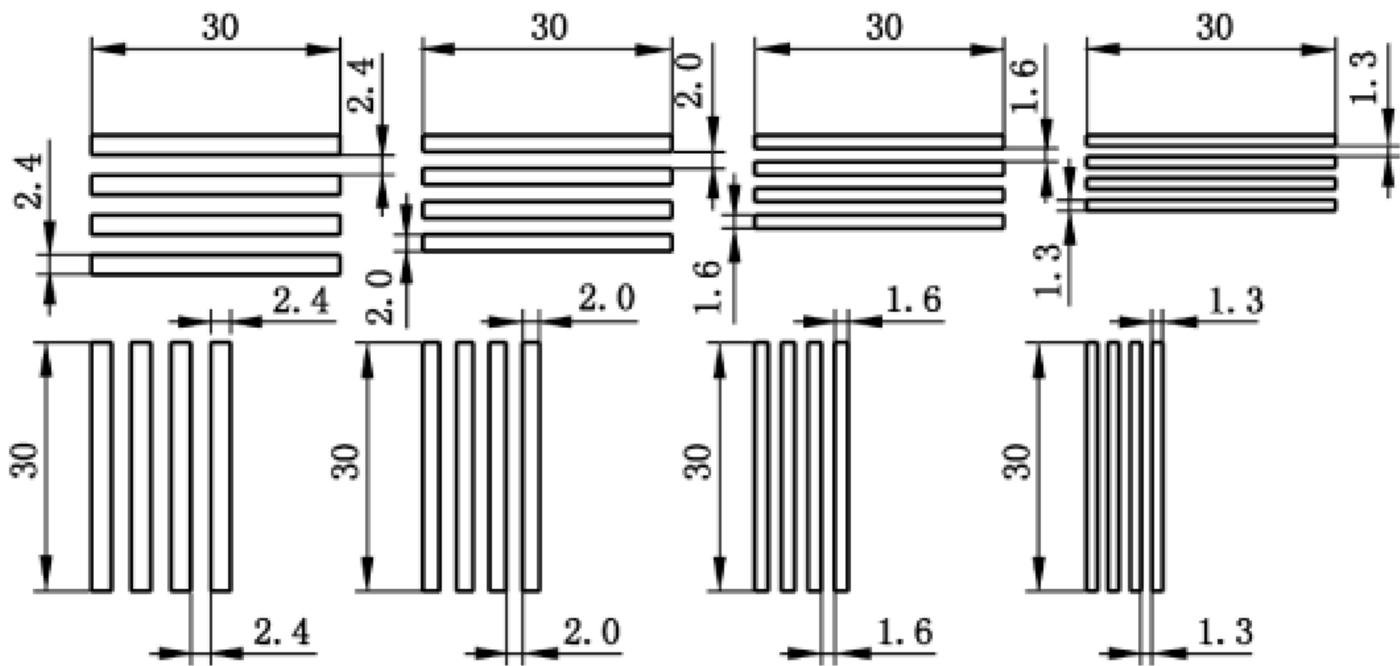
图 A.15 测试卡 3 尺寸图
